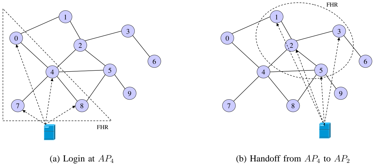
Fig. 5. FHR scheme.
