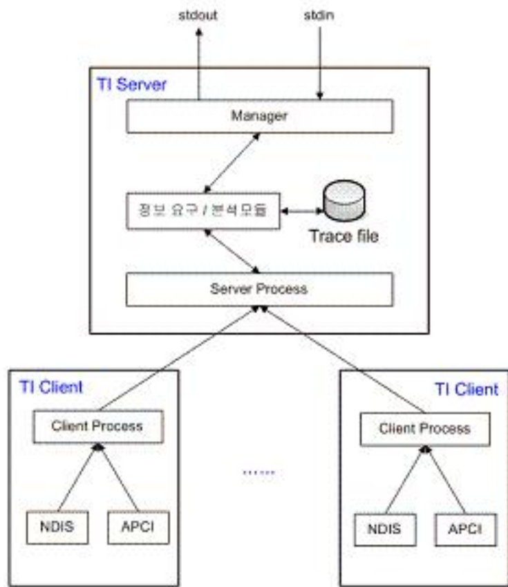
그림 4. TIS 전체 구조도
