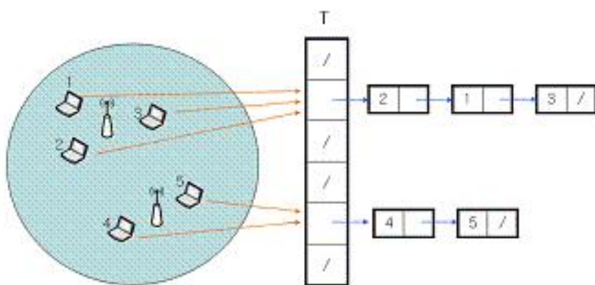
그림 7. 클라이언트 목록 관리
