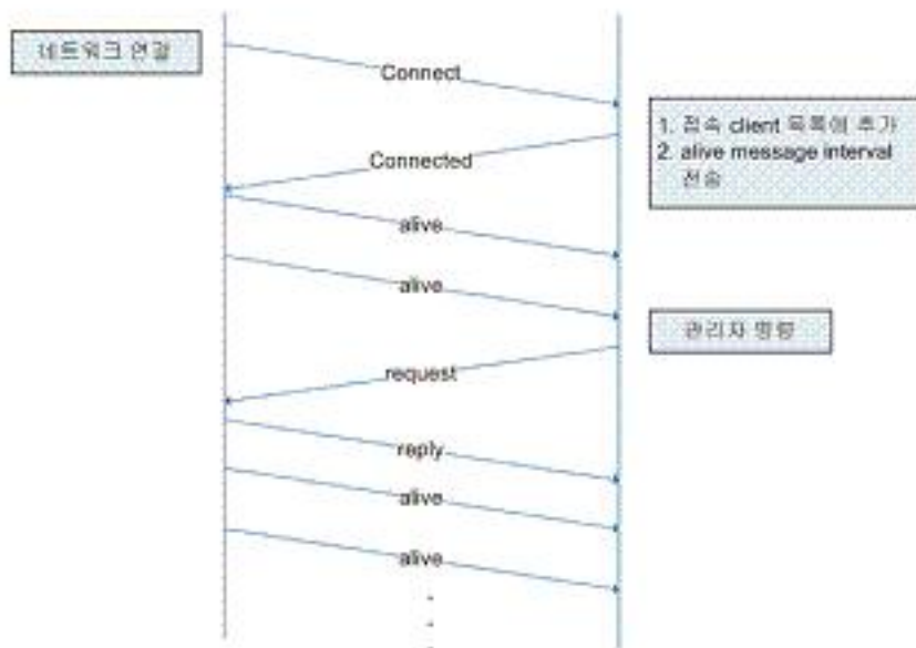
그림 5. TIS 클라이언트 / 서버 패킷 흐름도
