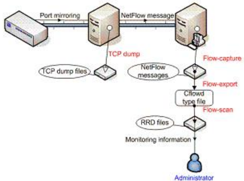
그림 2. 백본 라우터의 트래픽 측정
