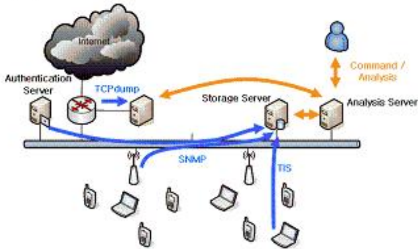
그림 1. NESPOT 사용 특성 분석을 위한 시스템 구조
